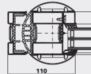
Porte anti-pince-doigts
