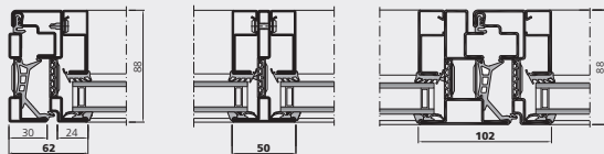
Fenêtre FB4
